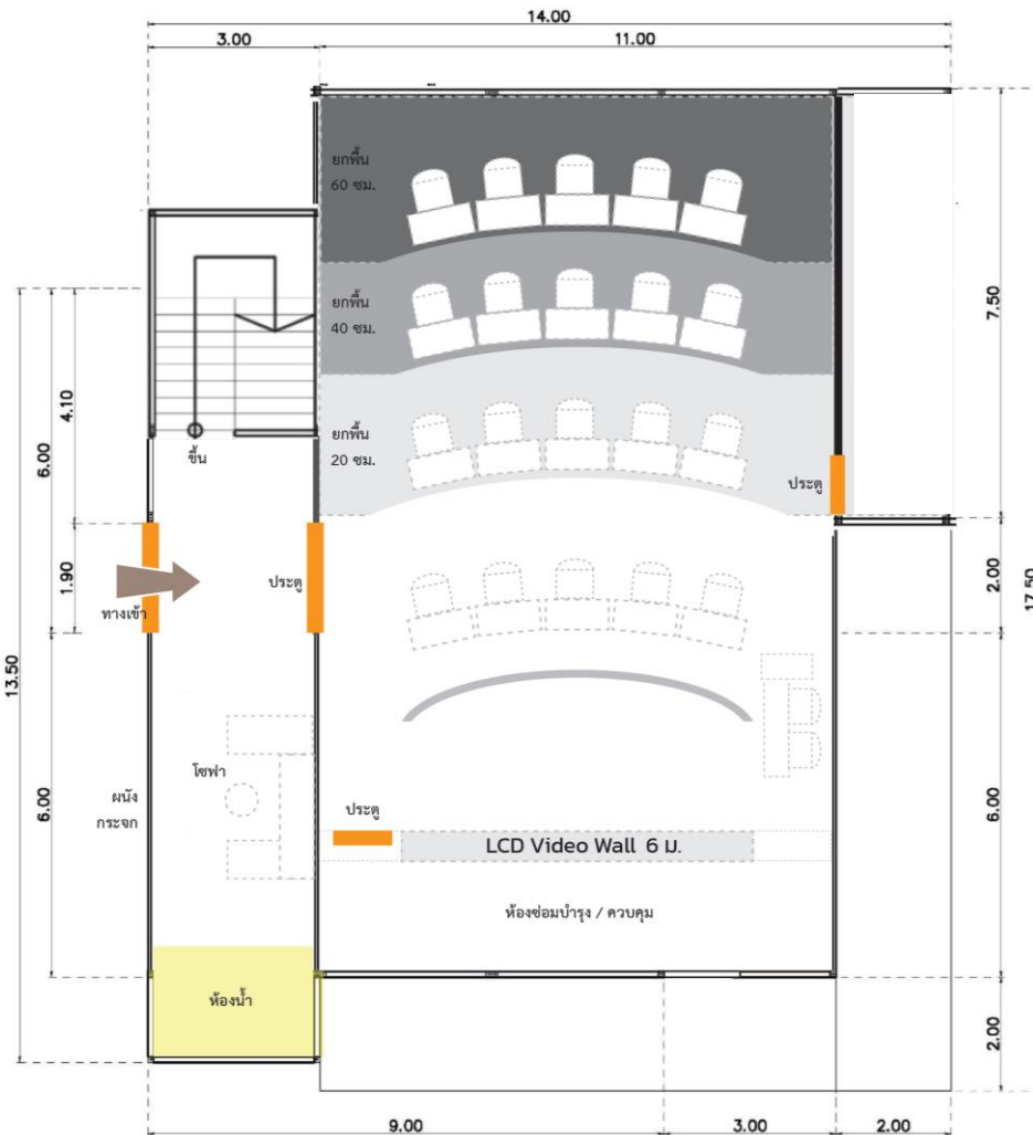
แผนผังชั้น 1 โซน Data Center พื้นที่ 200 ตรม.
