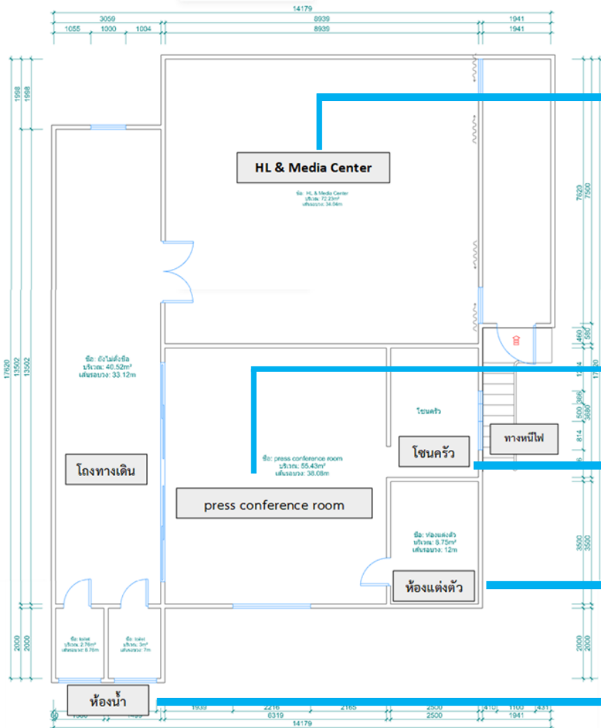
แผนผังชั้น 2 โซน HL พื้นที่ 200 ตรม.
